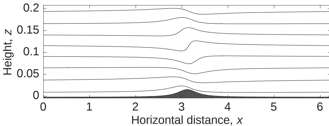
Streamfunction
